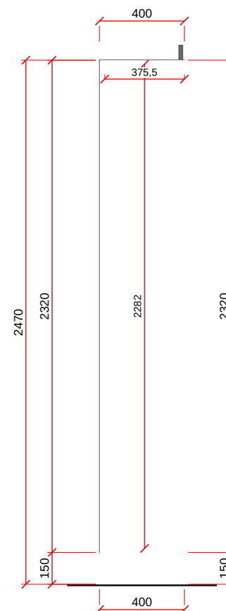
VISTA B - ESC. 1:25
