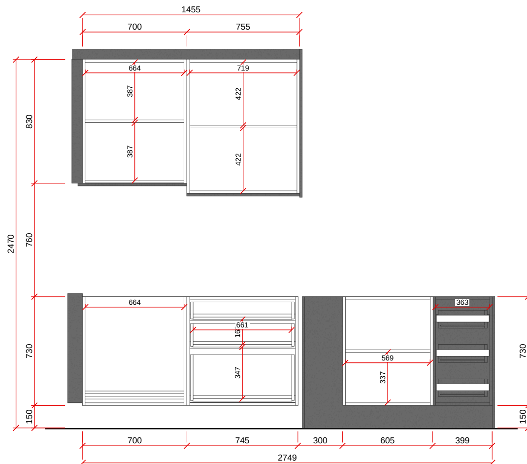
VISTA C - ESC. 1:25
