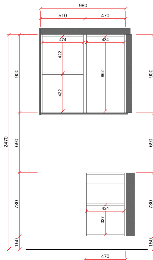
VISTA D - ESC. 1:25
